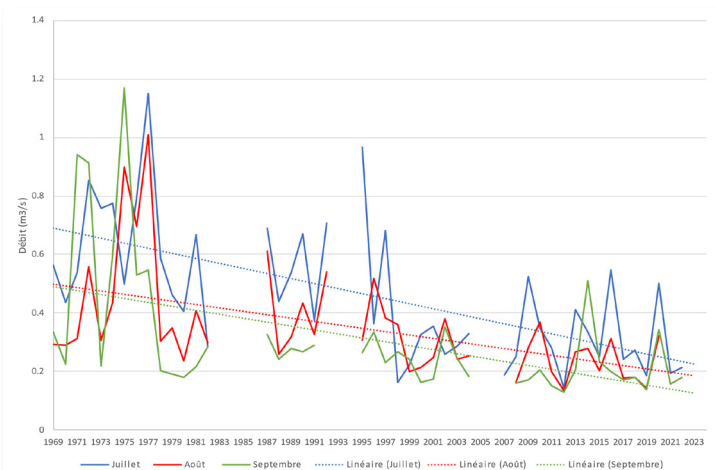
Débit moyen de la Têt mesuré à Serdinya (m 3 /s) et courbes de tendances. Le graphique ci-contre présente une absence de données sur plusieurs périodes. Mois juillet, août, septembre 1970-2022
